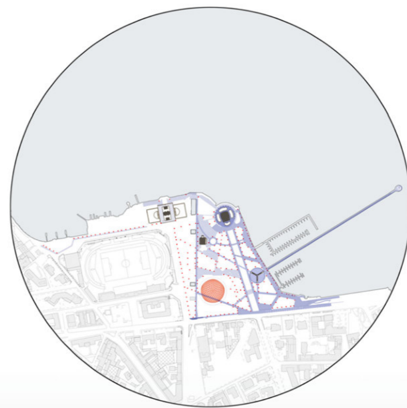
3. Percorsi - Illuminazione
